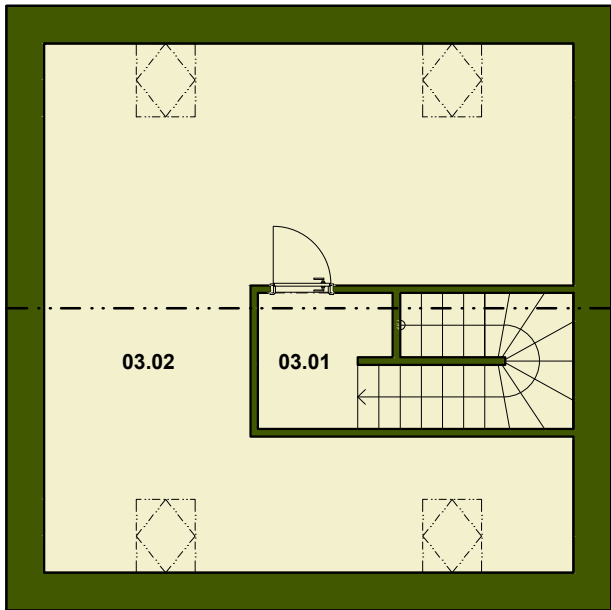
Půdorys podkroví
